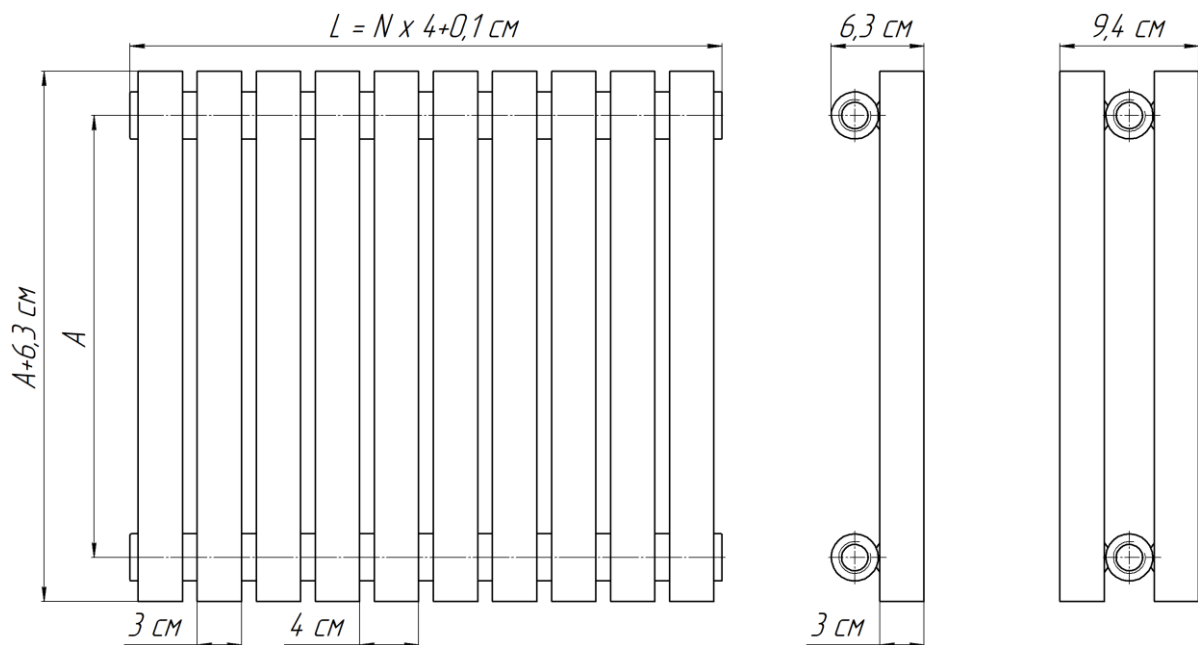
Рис 1. Радиатор «QUADRUM 30 V», где: А – межцентровый (монтажный) размер, см; N – количество секций; L – габаритная длина, см;
