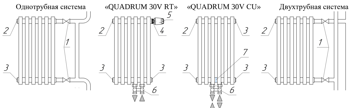
Рис.2 1. Вентиль. 2. Кран Маевского - воздухоотводчик. 3. Пробка глухая. 4. Встроенный термоклапан. 5. Термостатический элемент. 6. Запорно-присоединительный клапан. 7. Внутренняя перегородка.
